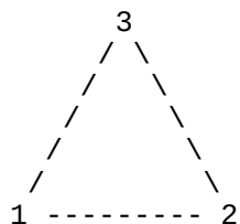
ESMF_MESHELEMENTTYPE_TRI
